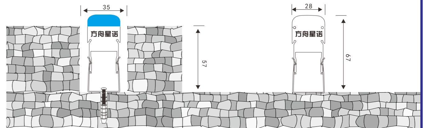
不锈钢弹片支架 (三)
