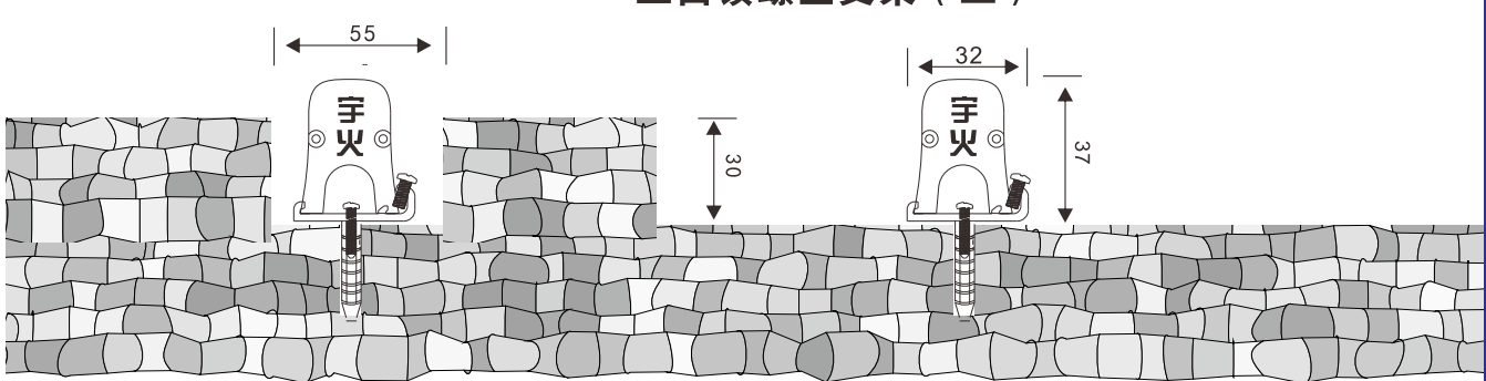
正面锁螺丝支架（三）
