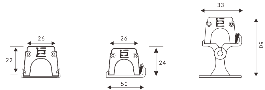
旋转支架（一）
