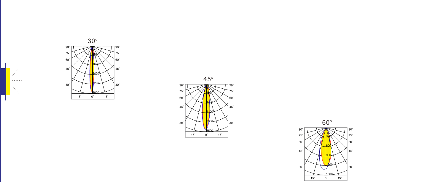
配光曲线
