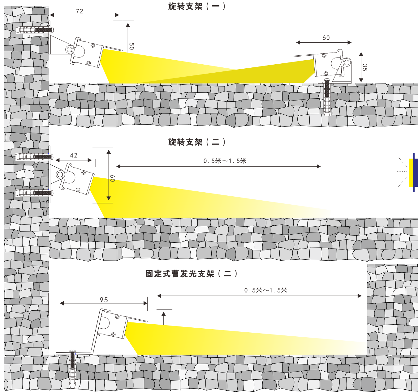
安装示意图
