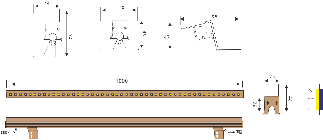
尺寸图
