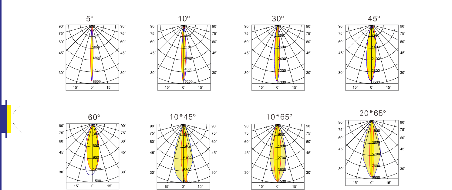
配光曲线
