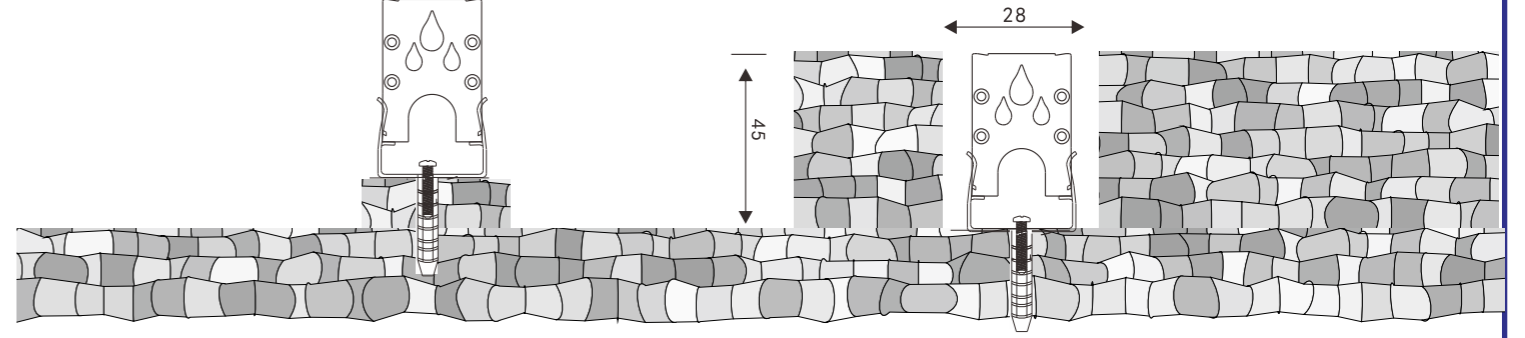
正面锁螺丝支架 (二)
