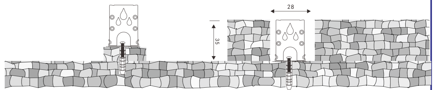
正面锁螺丝支架 (三)
